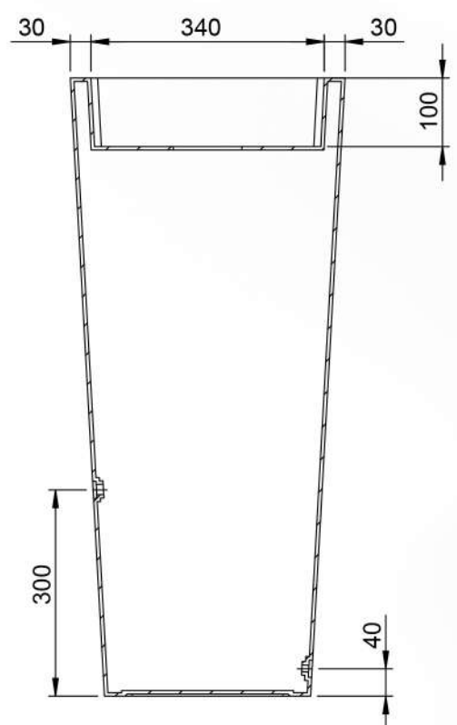
SECTION A-A
