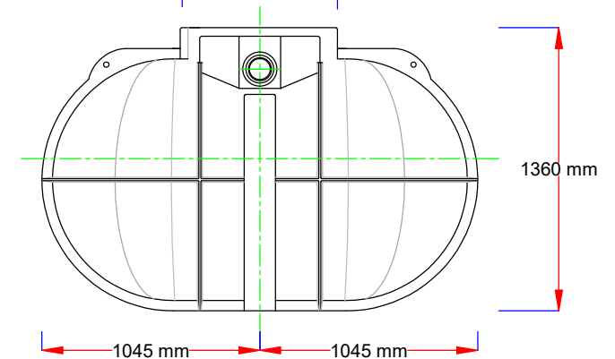
End elevation
