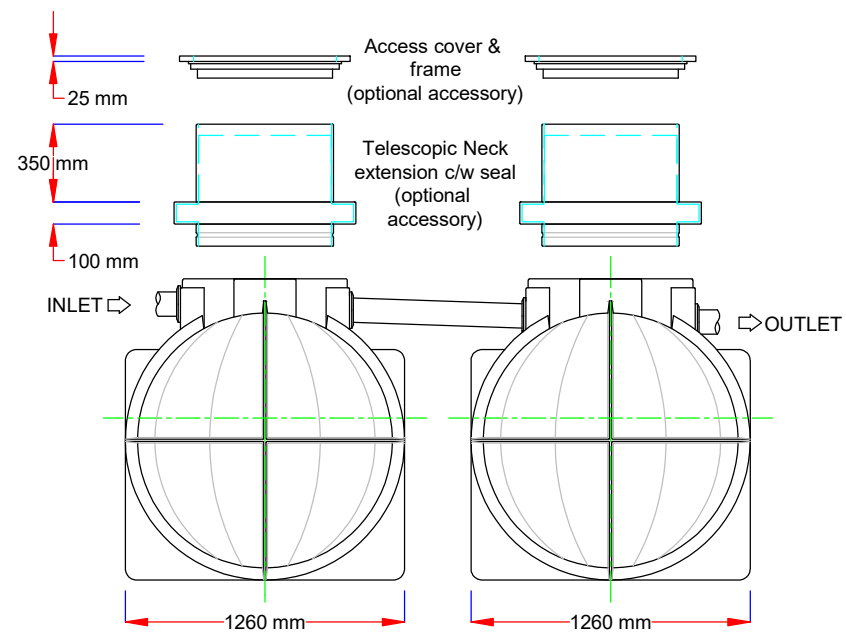
End elevation
