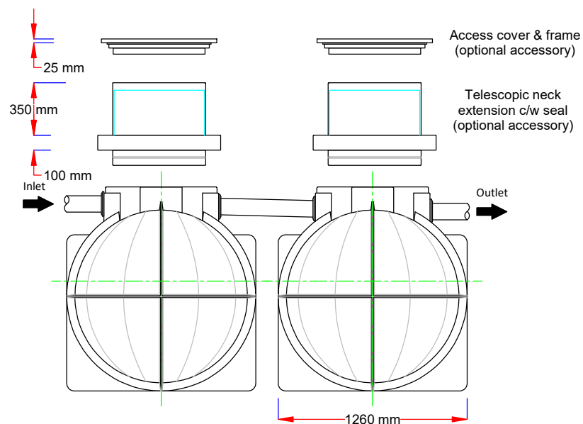
End elevation
