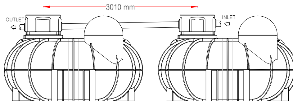
END ELEVATION
