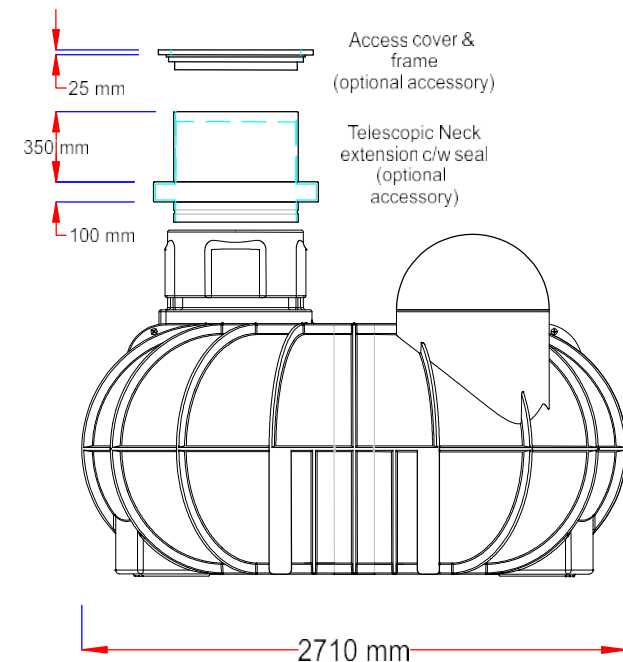
END ELEVATION
