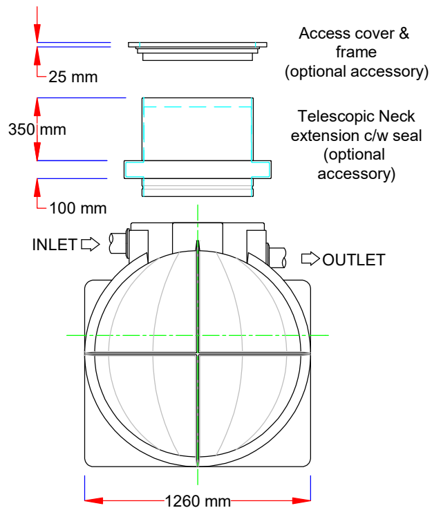
End elevation
