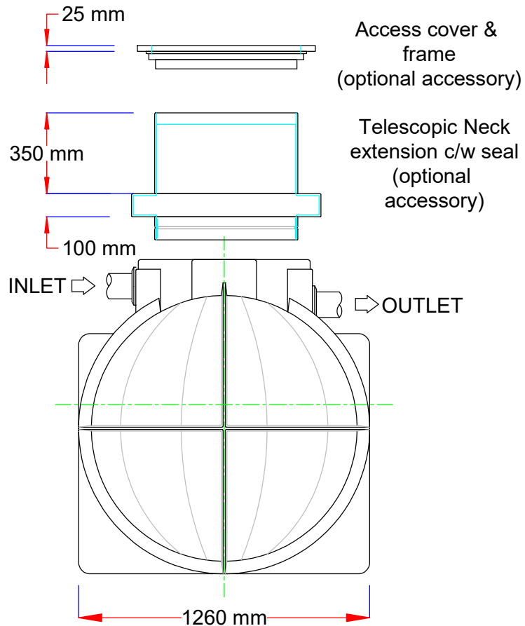
End elevation
