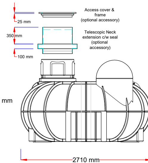
END ELEVATION
