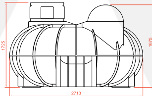
END ELEVATION
