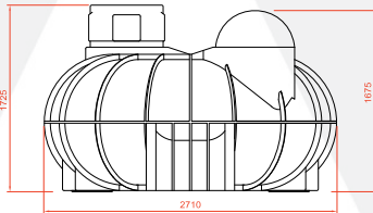
END ELEVATION
