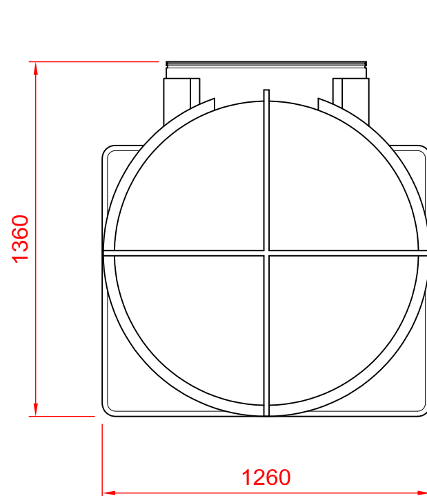
END ELEVATION
