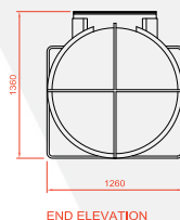
END ELEVATION
