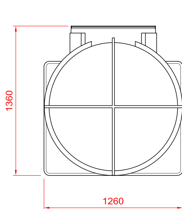
END ELEVATION
