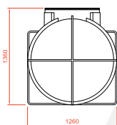
END ELEVATION
