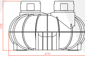
END ELEVATION
